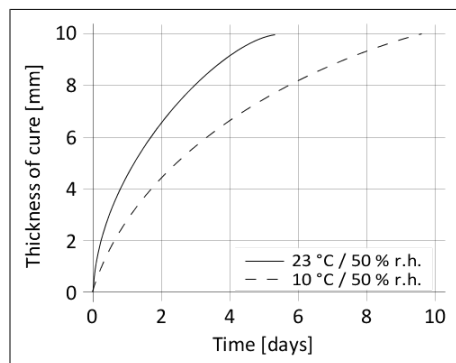
Diagramma 1: Velocità di indurimento per Sikaflex®-298 FC
