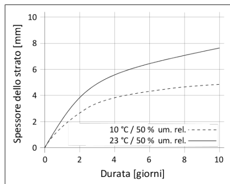
Diagramma 1: Velocità di indurimento per Sikaflex®-521 UV
