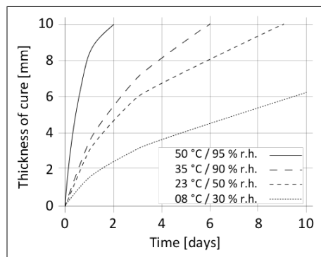
Grafico 1: Velocità di indurimento Sikasil® SG-20
