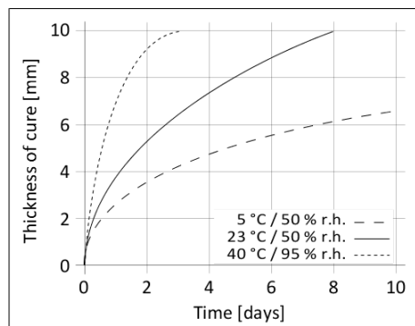
Grafico 1: Velocità di polimerizzazione Sikasil® WS-605 S
